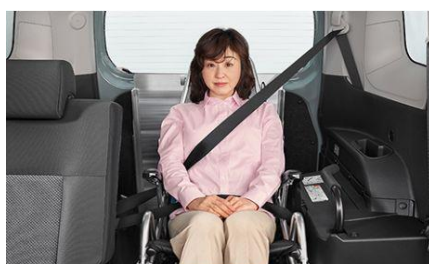
車いす用3点シートベルト
